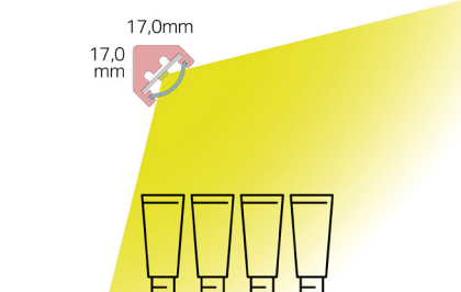
LED Leuchtenprofil 45° voll magnetisch
