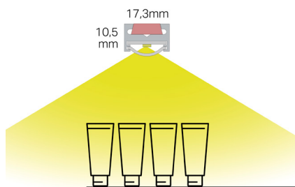
LED Leuchtenprofil 90° mit Funktionsnut
