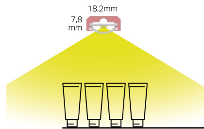
LED Leuchtenprofil 90° voll magnetisch filigran
