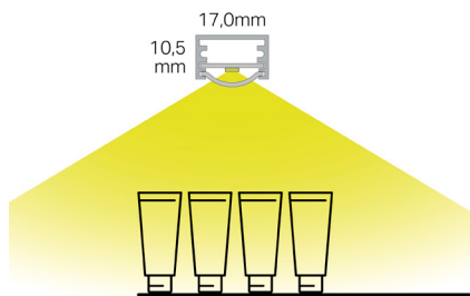
LED Leuchtenprofil 90°
